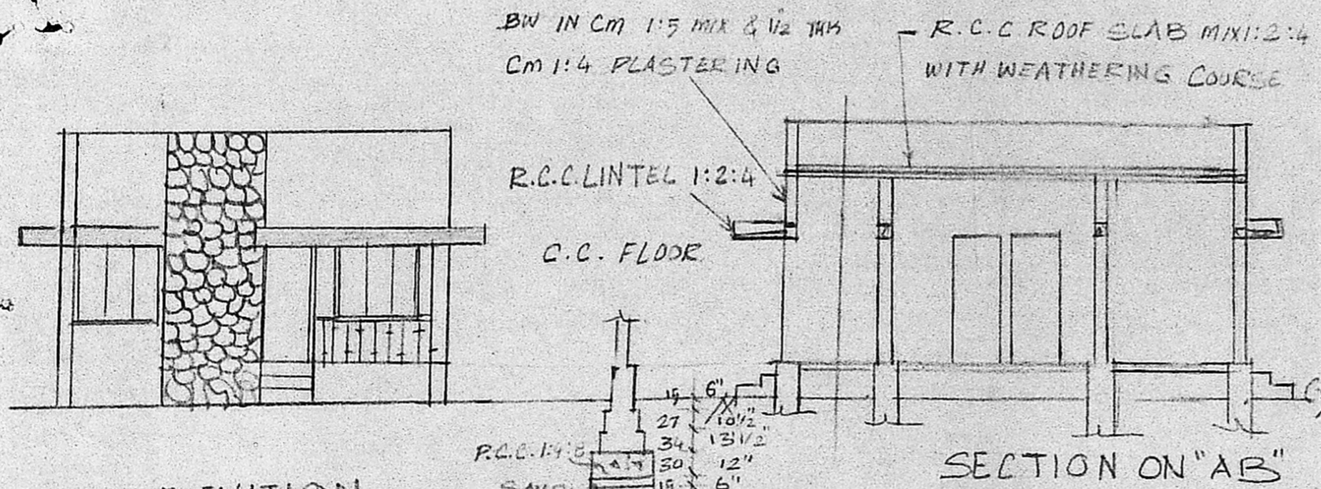
ELEVATION
